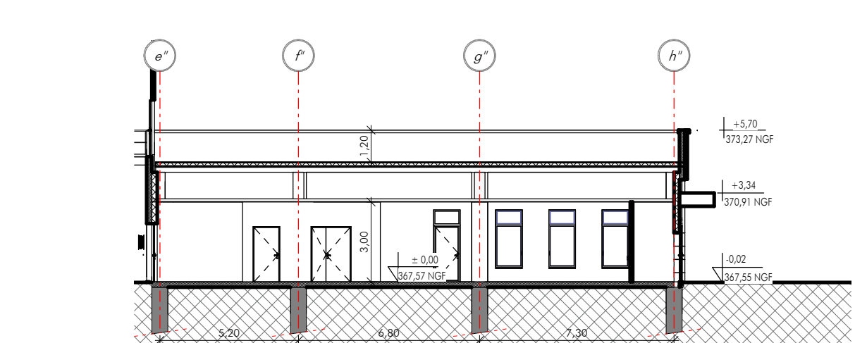
COUPE LONGITUDINALE K-K
