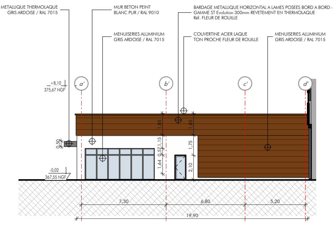
FACADE NORD-OUEST
