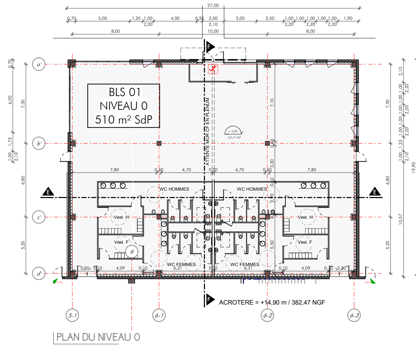
PLAN DU NIVEAU 0
