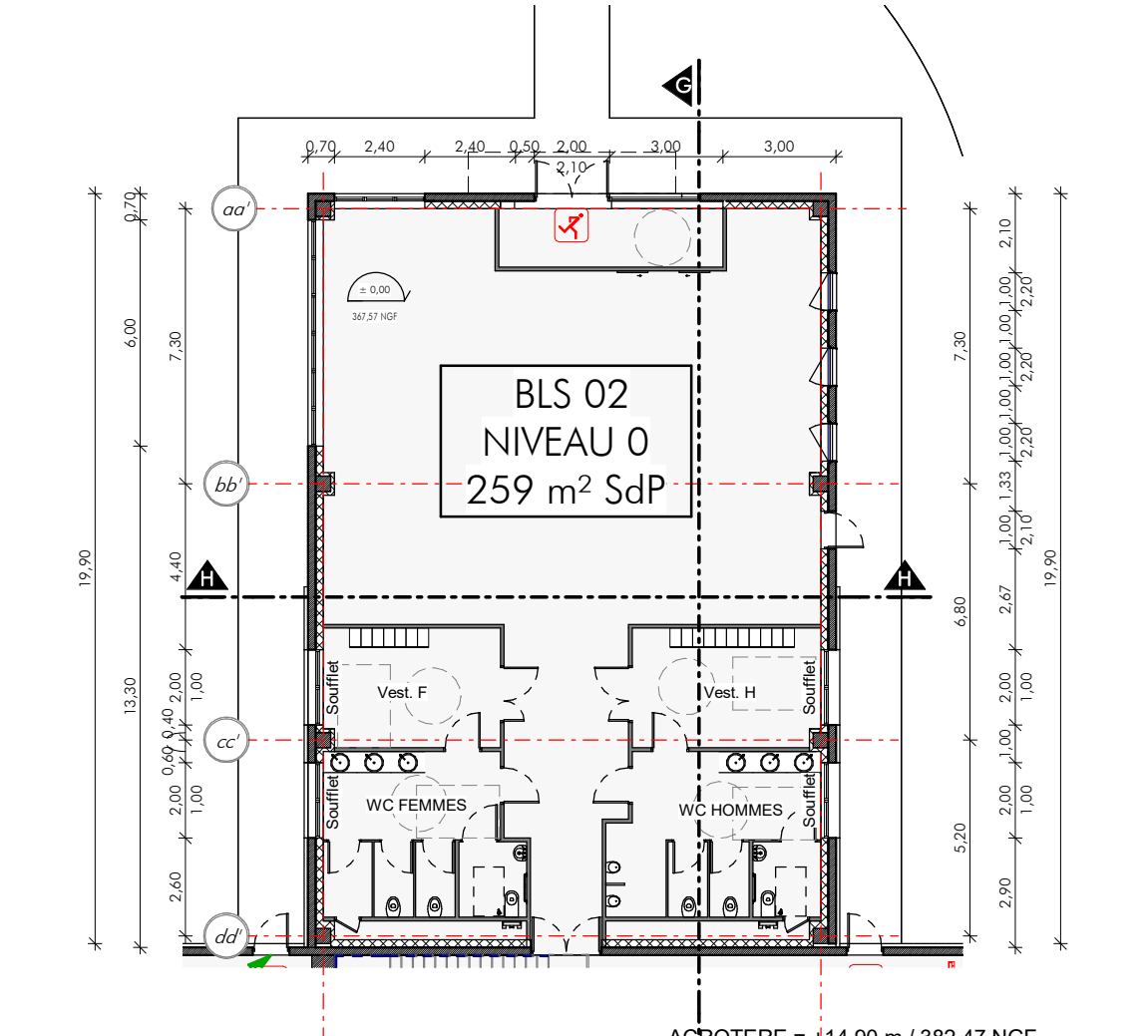
PLAN DU NIVEAU 0
