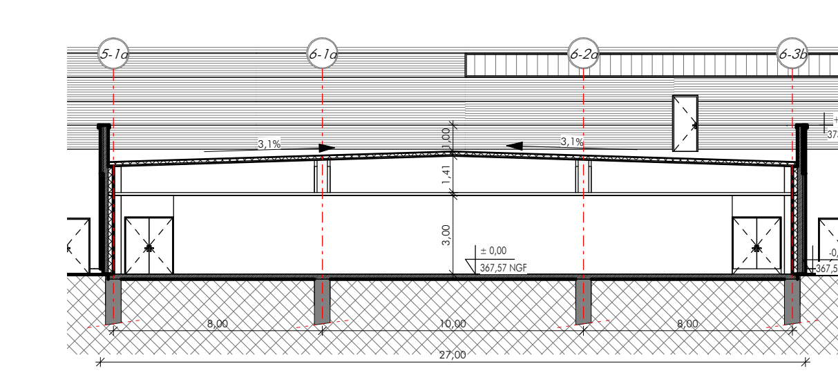
COUPE LONGITUDINALE I-I
