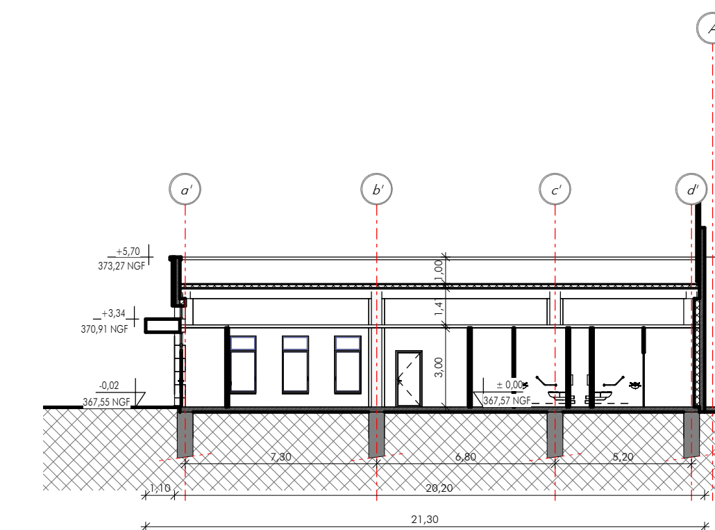
COUPE TRANSVERSALE F-F
