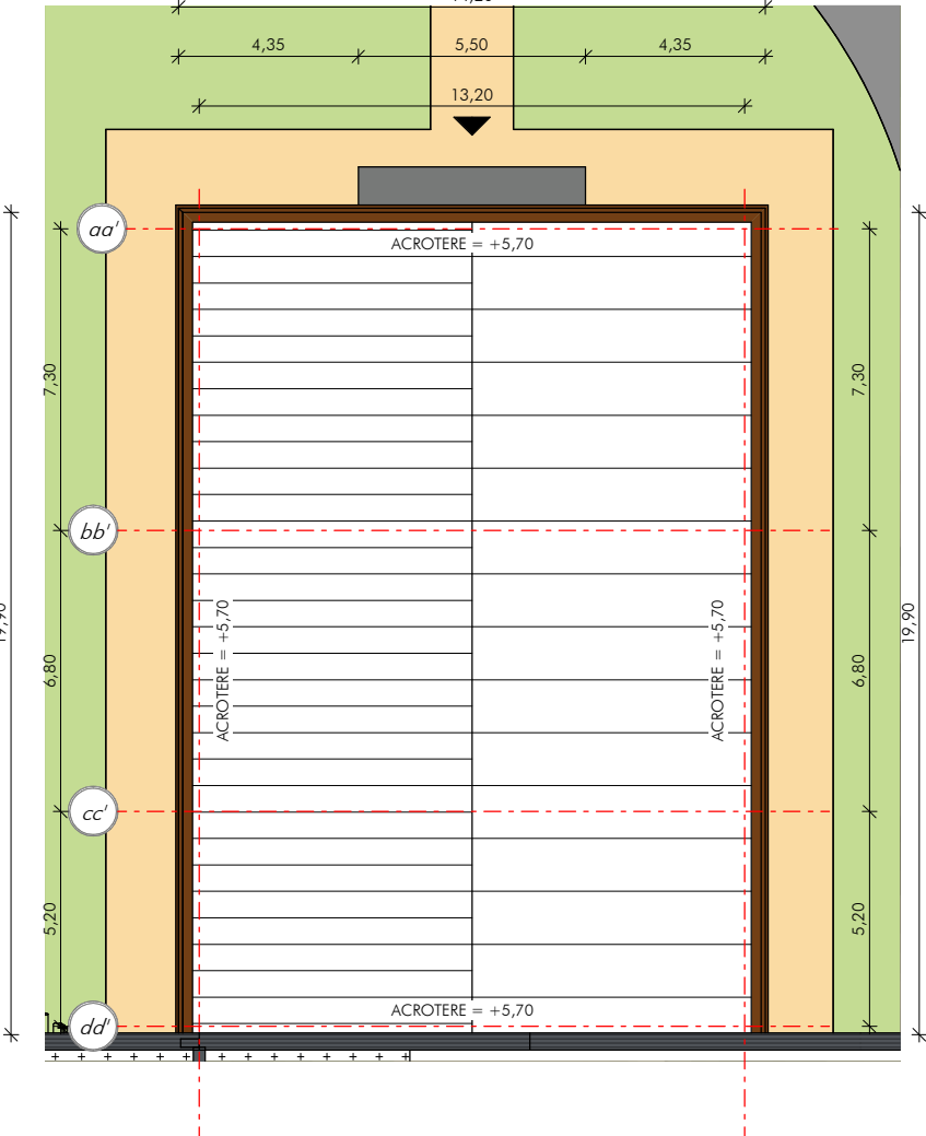
PLAN MASSE
