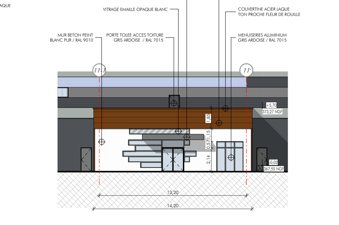
FACADE NORD-EST
