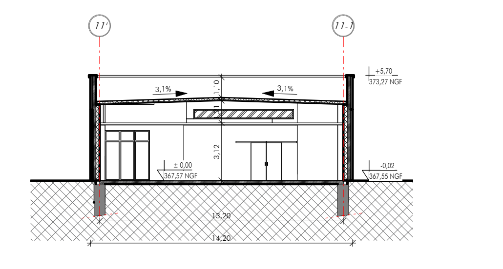
COUPE TRANSVERSALE H-H
