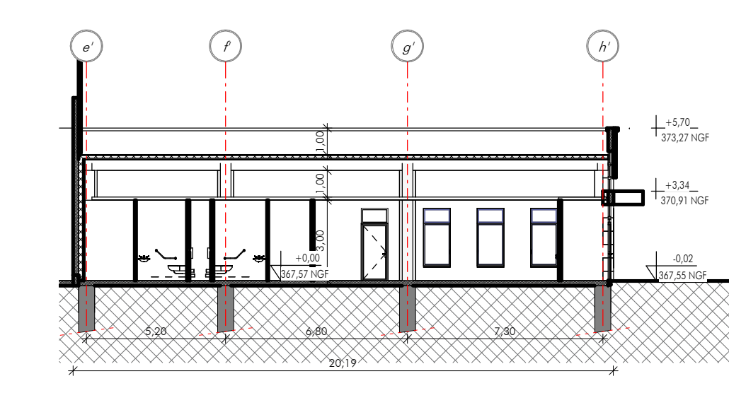
COUPE TRANSVERSALE J-J
