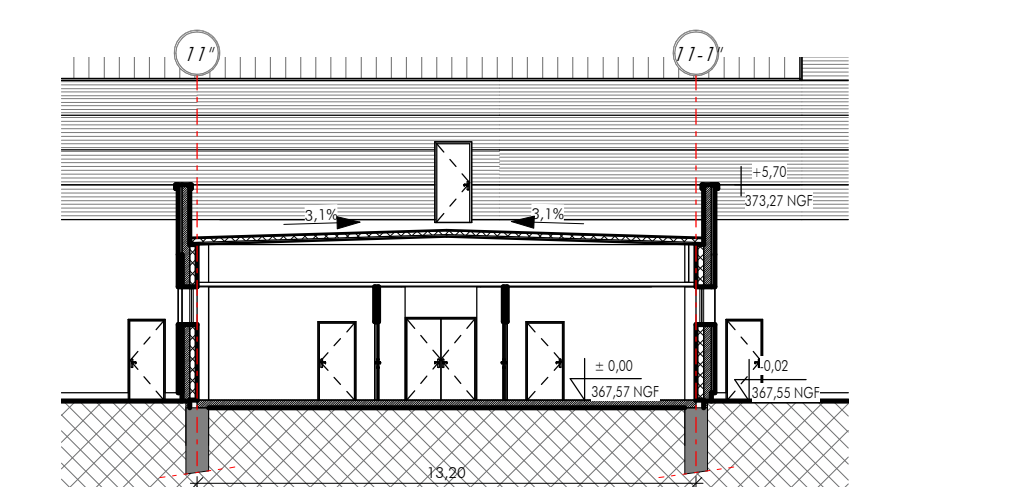
COUPE TRANSVERSALE L-L
