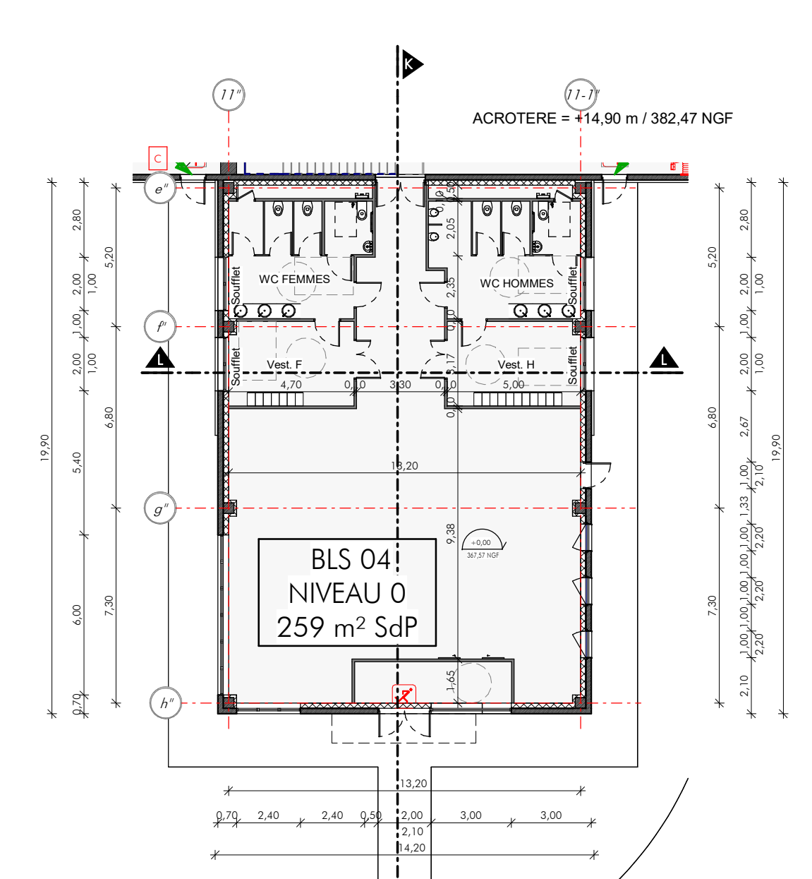
PLAN DU NIVEAU 0
