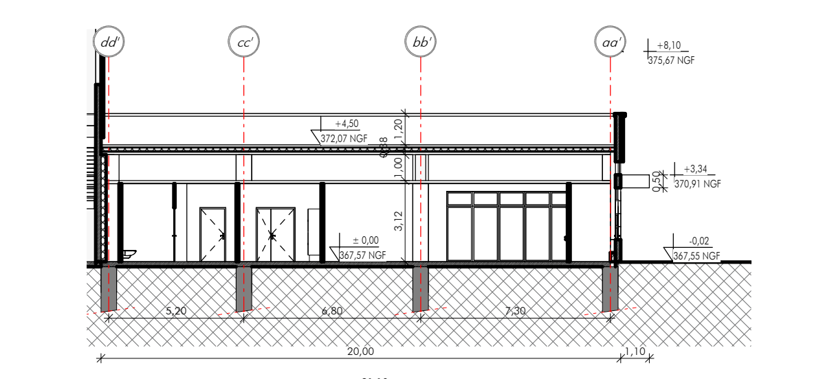
COUPE LONGITUDINALE B-B
