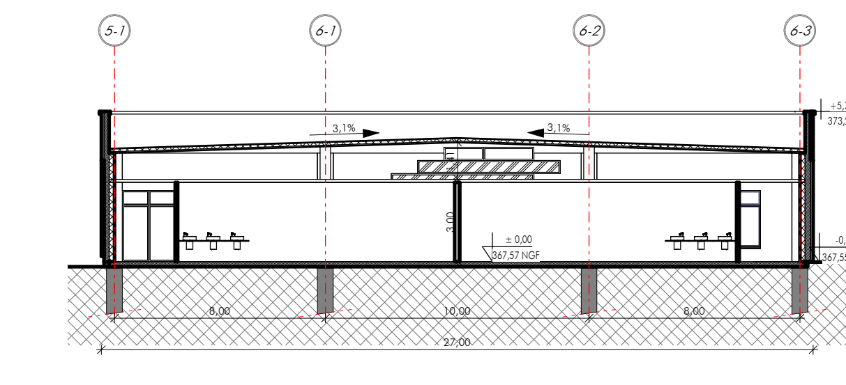
COUPE LONGITUDINALE E-E
